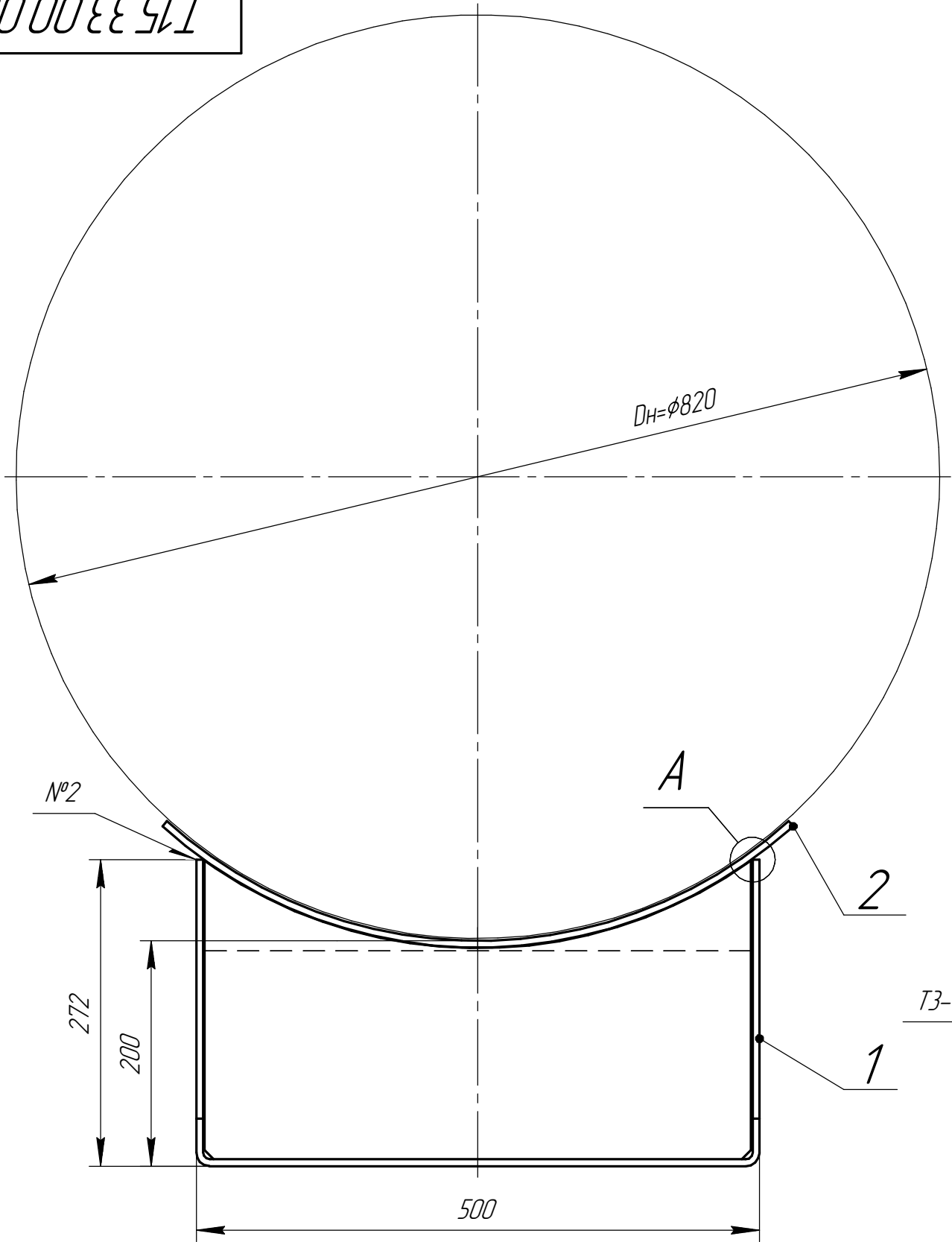
Дет. поз. 1 (1:10)
