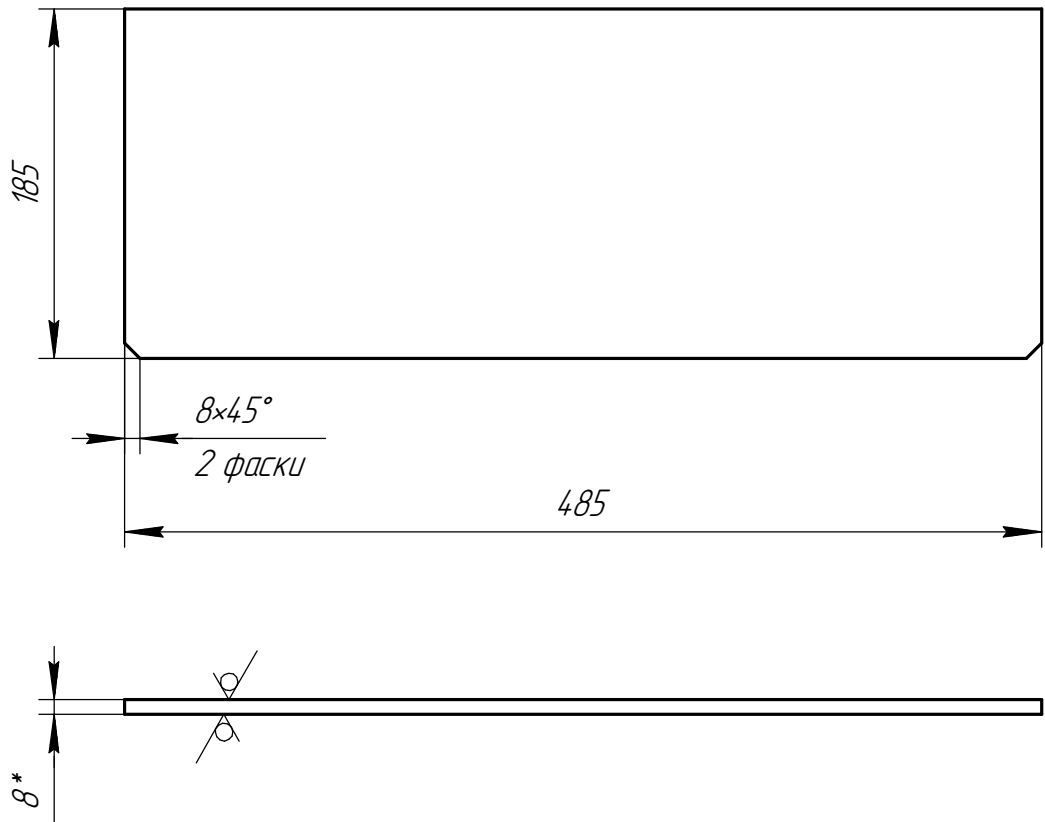
Дет. поз. 4 (1:4)
