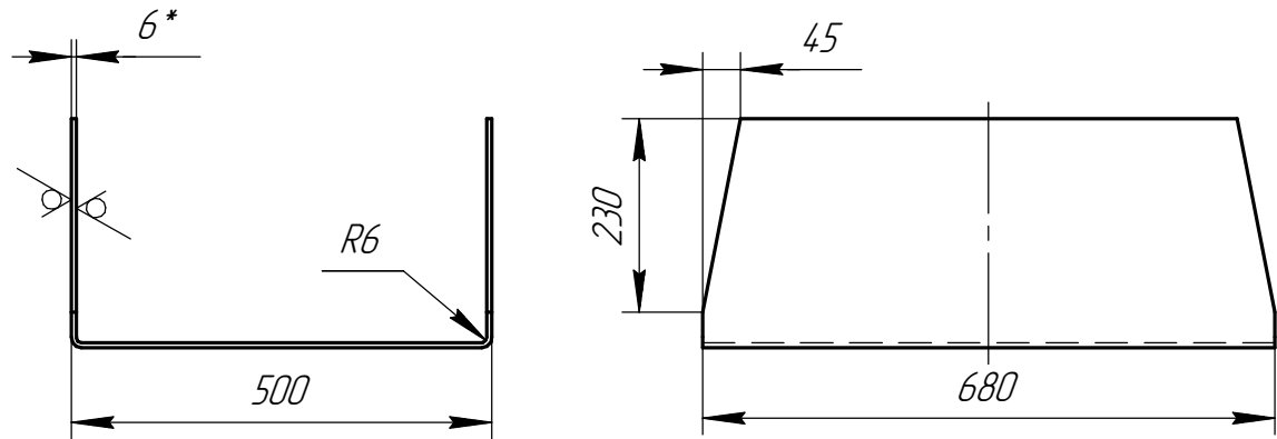
Дет. поз. 1 (1:10)
